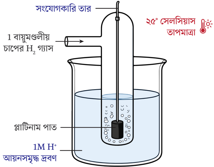
চিত্রঃ প্রমাণ হাইড্রোজেন তড়িৎদ্বারের গঠন
