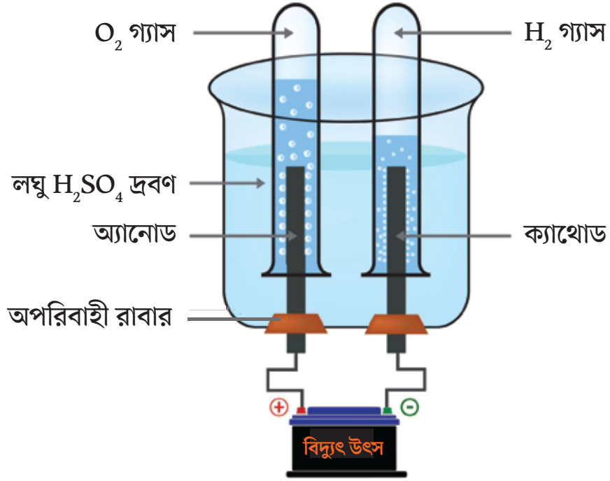
চিত্রঃ লঘু সালফিউরিক এসিড মিশ্রিত পানির তড়িৎ বিশ্লেষণ
