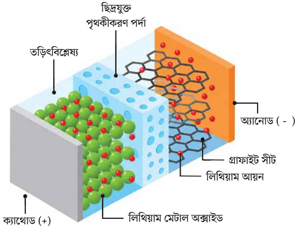
চিত্রঃ লিথিয়াম আয়ন ব্যাটারির গঠন।
